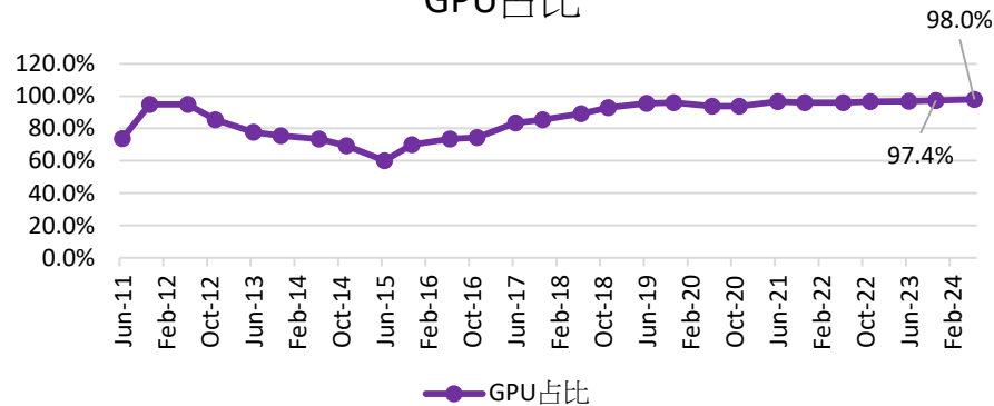
GPU占比
